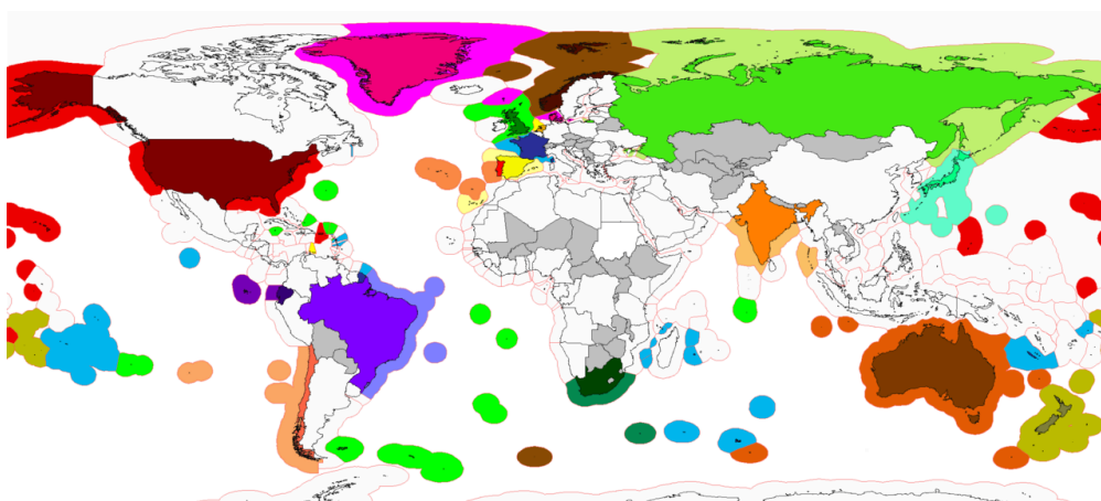
Страны с наиболее удаленными ИЭЗ
