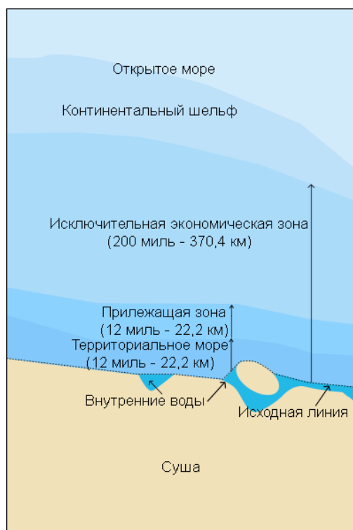
Морские зоны в соответствии с Конвенцией ООН по морскому праву
